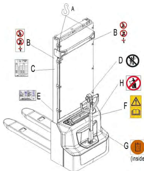
Fig.3 :Étiquettes de sécurité et d'avertissement
