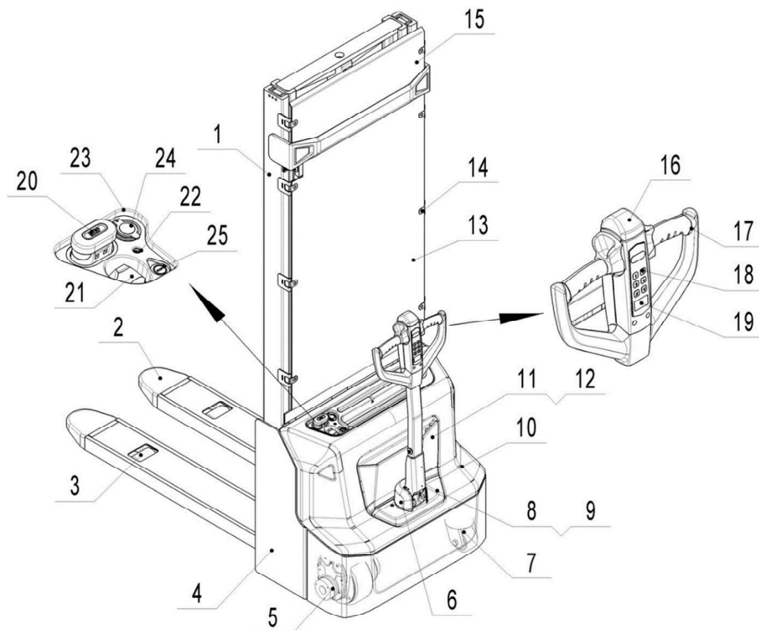
Fig. 1 : Vue d'ensemble des principaux éléments
