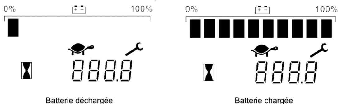
Fig. 13 : Indicateur de décharge de la batterie
