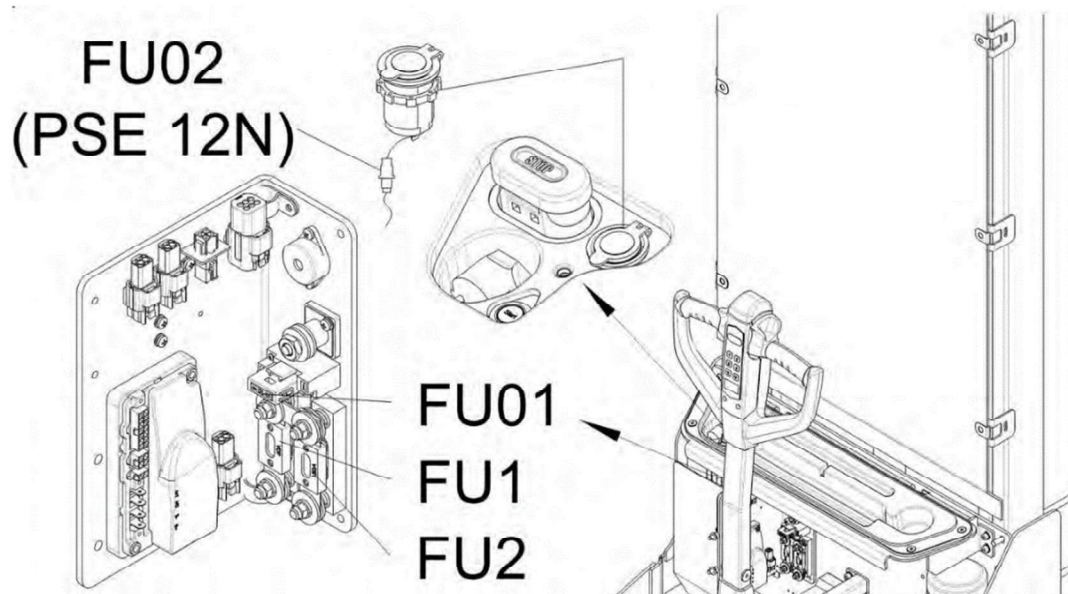
Fig. 15 : Emplacement des fusibles
