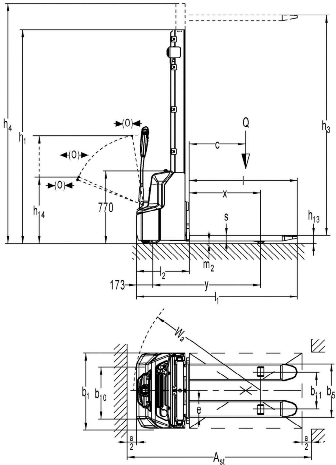
Fig. 2 : Données techniques
