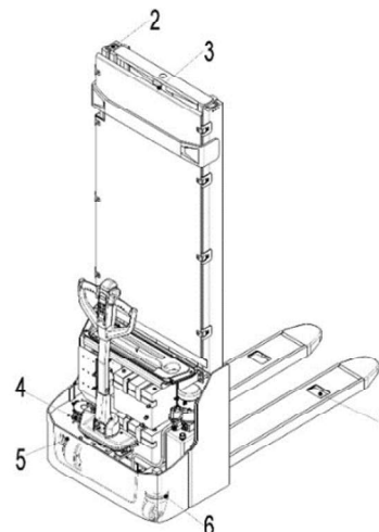
Fig. 14 : Points de graissage
