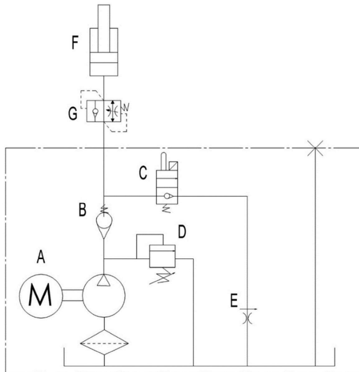
Fig. 18 : Circuit hydraulique
